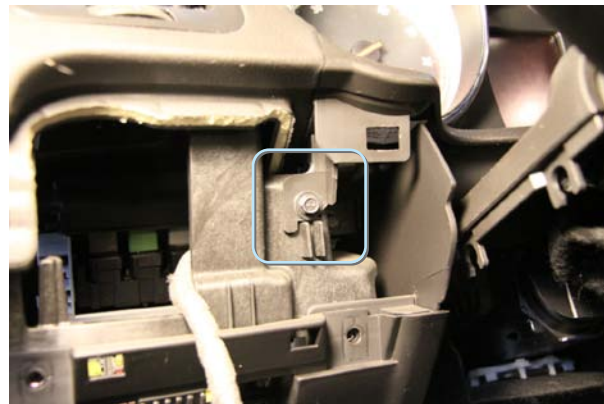
Фото 1.10. Крепление подторпедника
